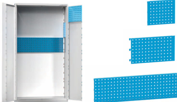
Panel perforovaný do bočnice – 2 ks
